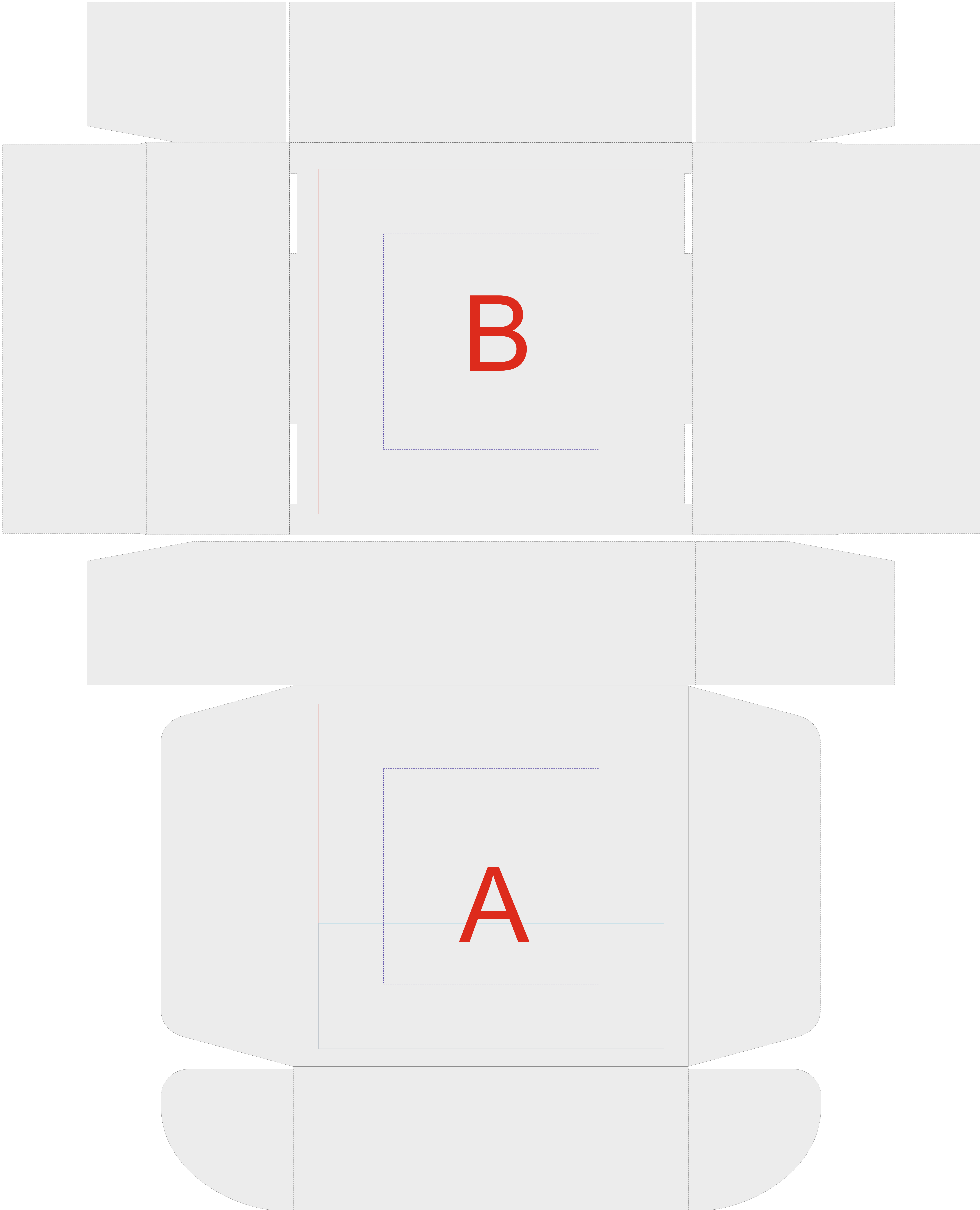
Коробка в разложенном виде ВНЕШНЯЯ СТОРОНА
